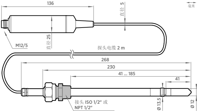
DMP8 尺寸
