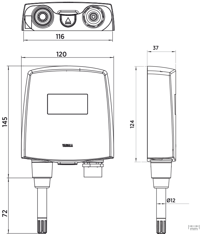
变送器尺寸
