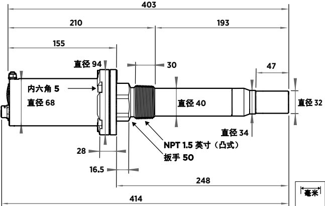
MGP262 尺寸
